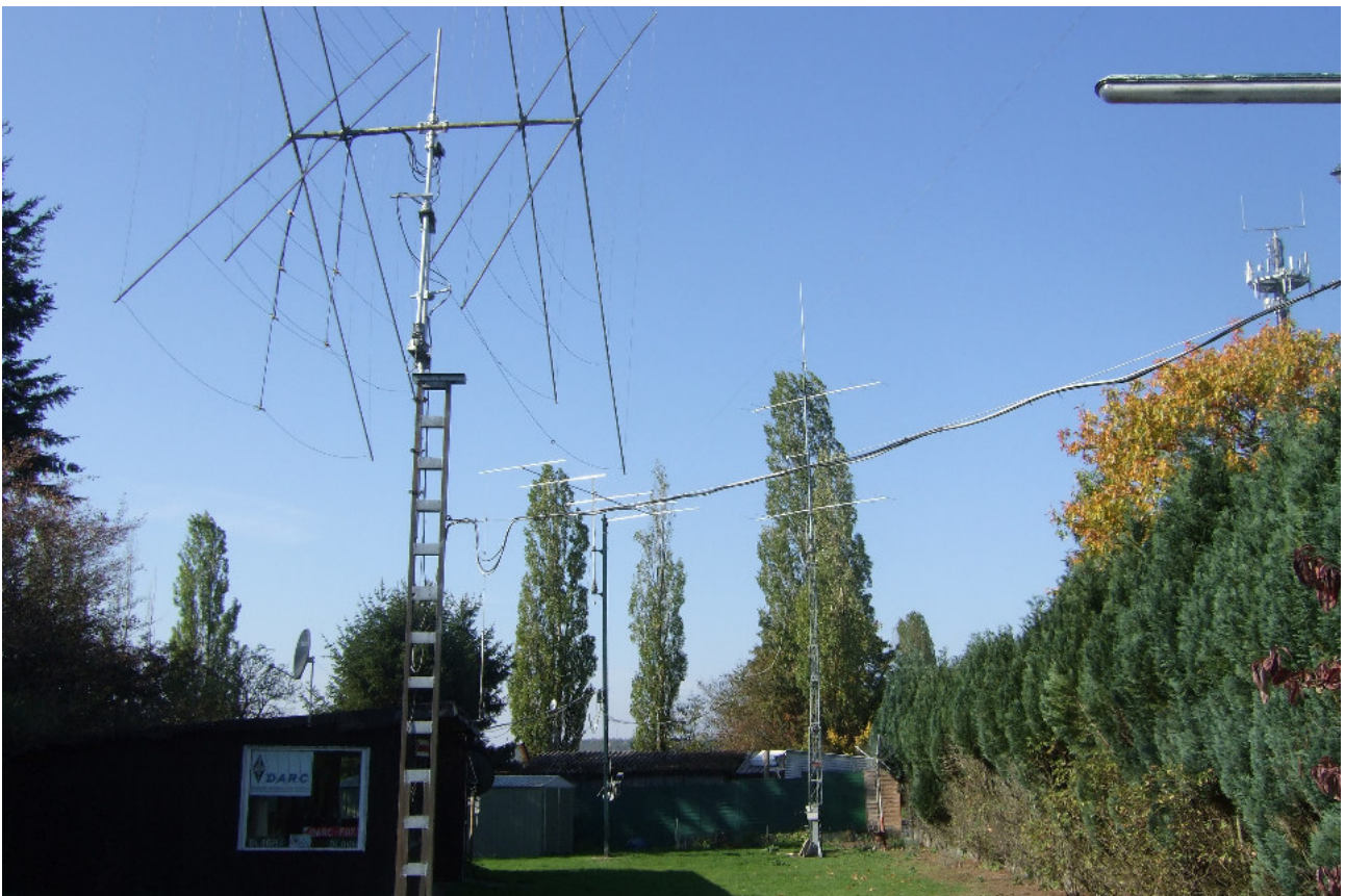
Antennen 2 EL Quad 20-10 Meter, 5EL Yagi für 50 Mhz, 2 x 13 EL Yagis für 144 Mhz
